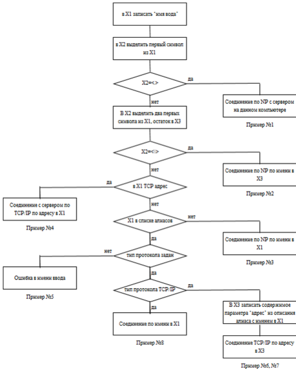
Блок-схема присоединений
