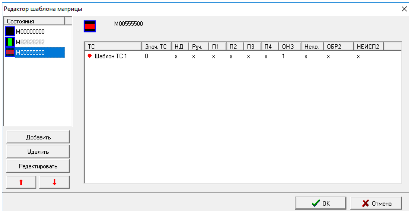
Окно описания шаблона матрицы ('темный' щит)
